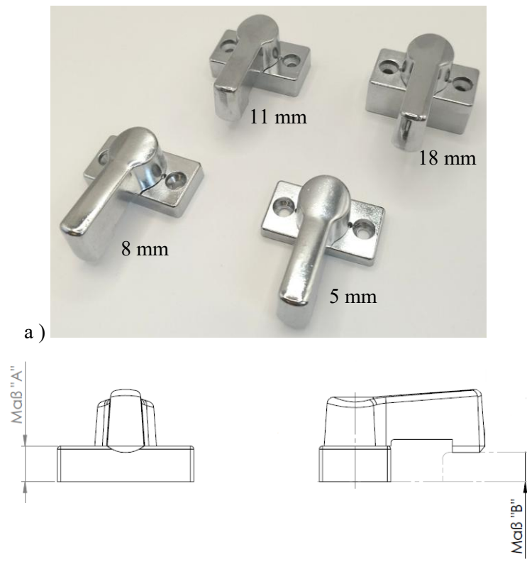
Abbildung 2: Die vier Höhen des Vorreibers TÜRVERBINDUNGSRIEGEL 5100
