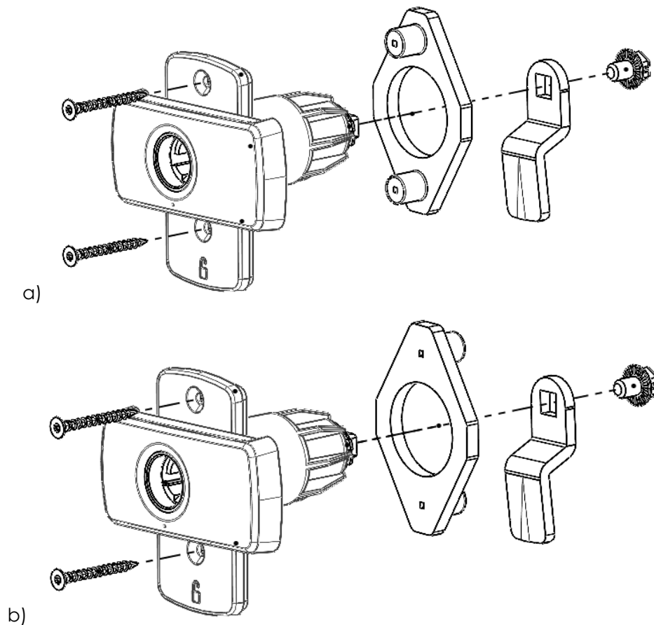
Abbildung 4: Montage des Kompressionsverschlusses SLIM LINE 2018 mit Schrauben und den optionalen Artikeln, a) mit versenkten Dornen der Montageplatte und b) nicht versenkten Dornen der Montageplatte
