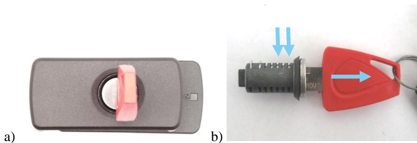
Abbildung 6: Demontage des SCS 53er-Schließzylinders im Kompressionsverschluss SLIM LINE 2018 mit a) Ausgangsposition und b) Entfernung des Demontageschlüssels
