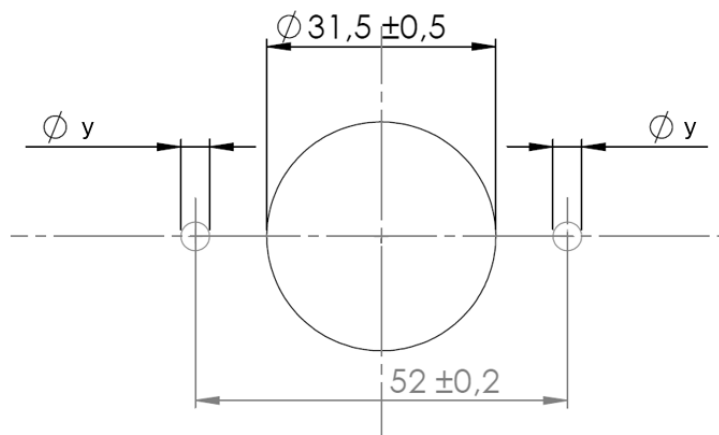
Abbildung 3: Einbaumaße für Kompressionsverschluss SLIM LINE 2018
