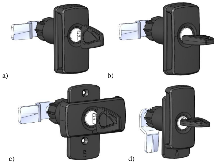
Abbildung 8: Kompressionsverschluss SLIM LINE 2018 a) im geschlossenen und komprimierten Zustand, b) im aufgeschlossen und komprimierten, c) im dekomprimierten Zustand und d) im geöffneten Zustand
