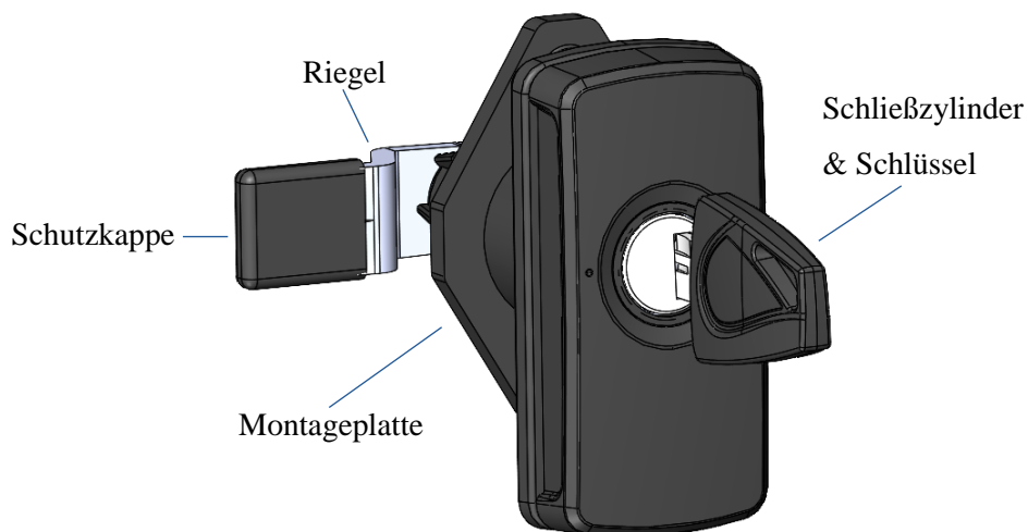
Abbildung 1: Kompressionsverschluss SLIM LINE 2018
