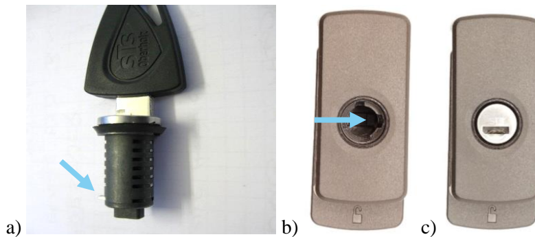
Abbildung 5: Einsetzen des SCS 53er-Schließzylinders im Kompressionsverschluss SLIM LINE 2018 mit a) Ausgangsposition, b) Ausrichtung des Verschlusses und c) Endposition
