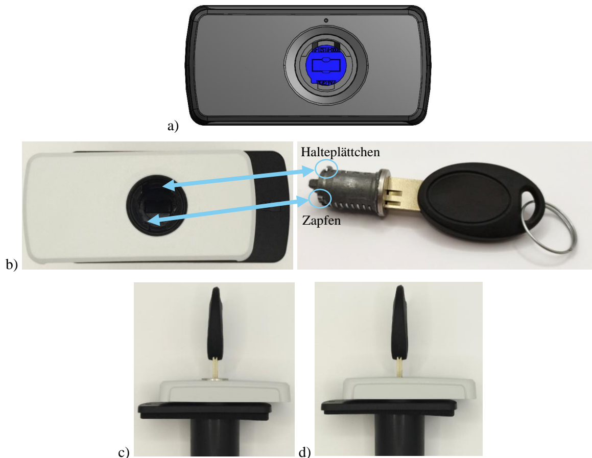
Abbildung 7: Montage eines HSC-Schließzylinders mit a) Mitnehmer b) den beiden Sicherungspunkten, c) vor Einrasten und d) nach Einrasten des Schließzylinders
