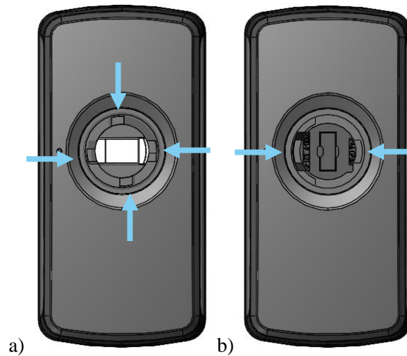
Abbildung 2: Kompressionsverschluss SLIM LINE 2018 vorgerichtet für a) STS- / Zadi Schließzylinder und b) HSC- / FF2-Schließzylinder
